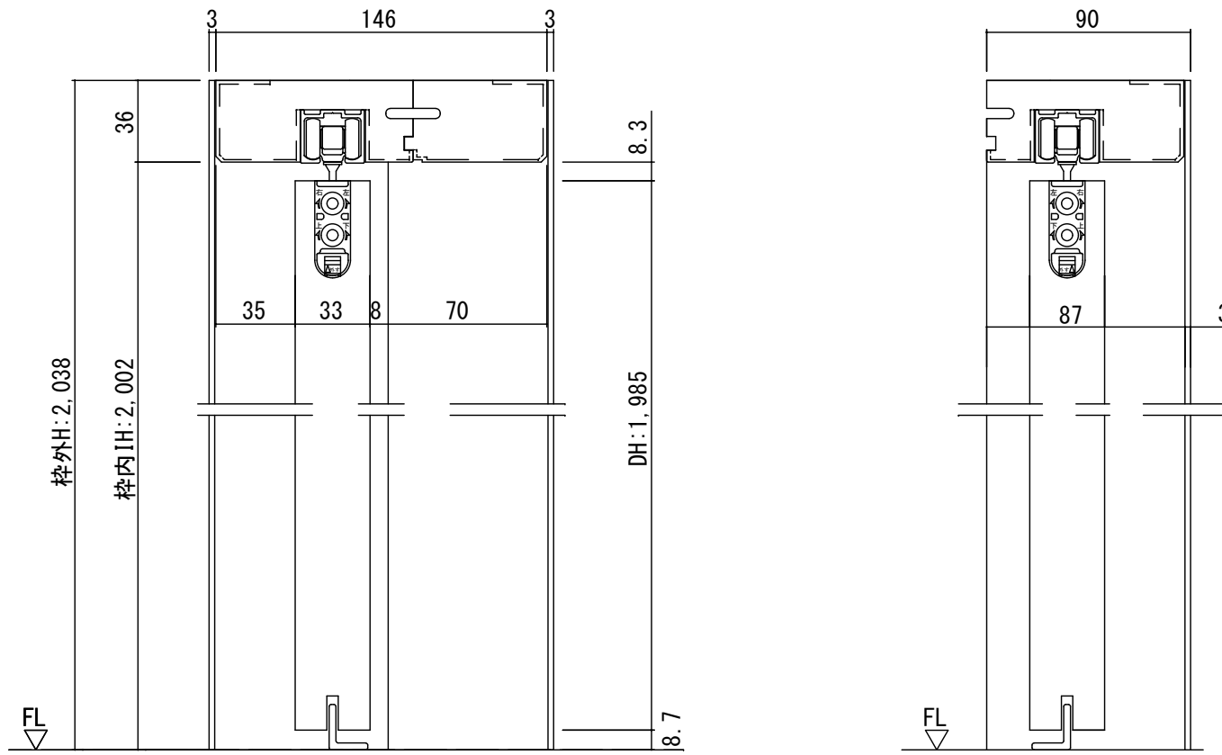
断面図
